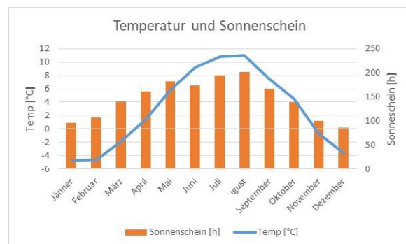
Abbildung 8: Durchschnittstemperaturen (blaue Linie) und Sonnenscheindauer jeweils 1990-2020 beim Watzmannhaus (1923 m ü. NHN).
