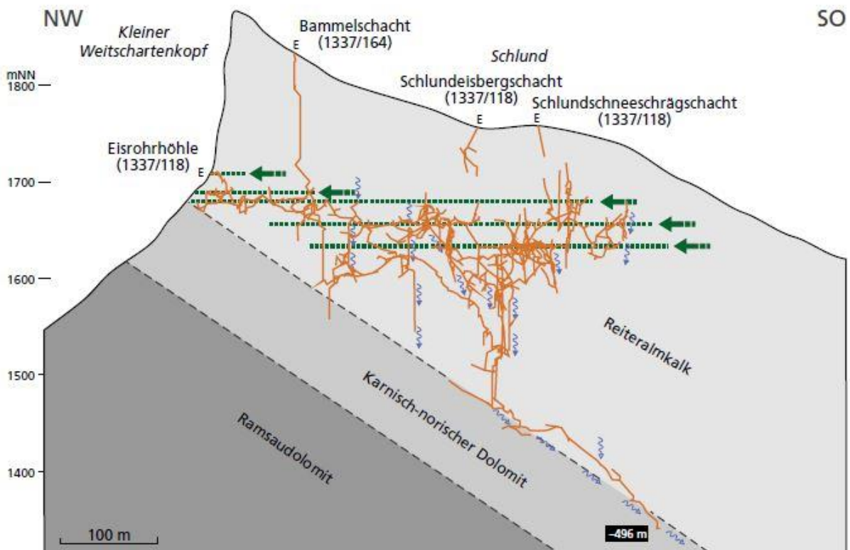
Abbildung 9: Aufriss des Eisrohrhöhle-Bammelschacht-Systems von NW nach SO (Quelle: Wisshak et al. 2013; Wiedergabe mit Genehmigung)
